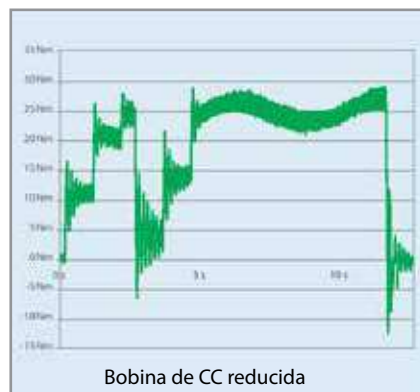
Los convertidores con bobinas de CC reducidas generan niveles armónicos más altos, especialmente en los intervalos de frecuencia más elevados.
