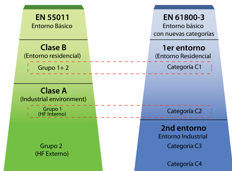
Comparación de niveles de interferencia
