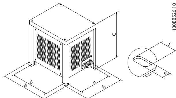
Ilustración 5.6 IP23 con montaje en suelo
