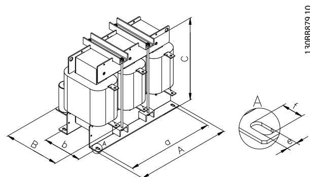
Ilustración 5.7 IP00 con montaje en suelo
