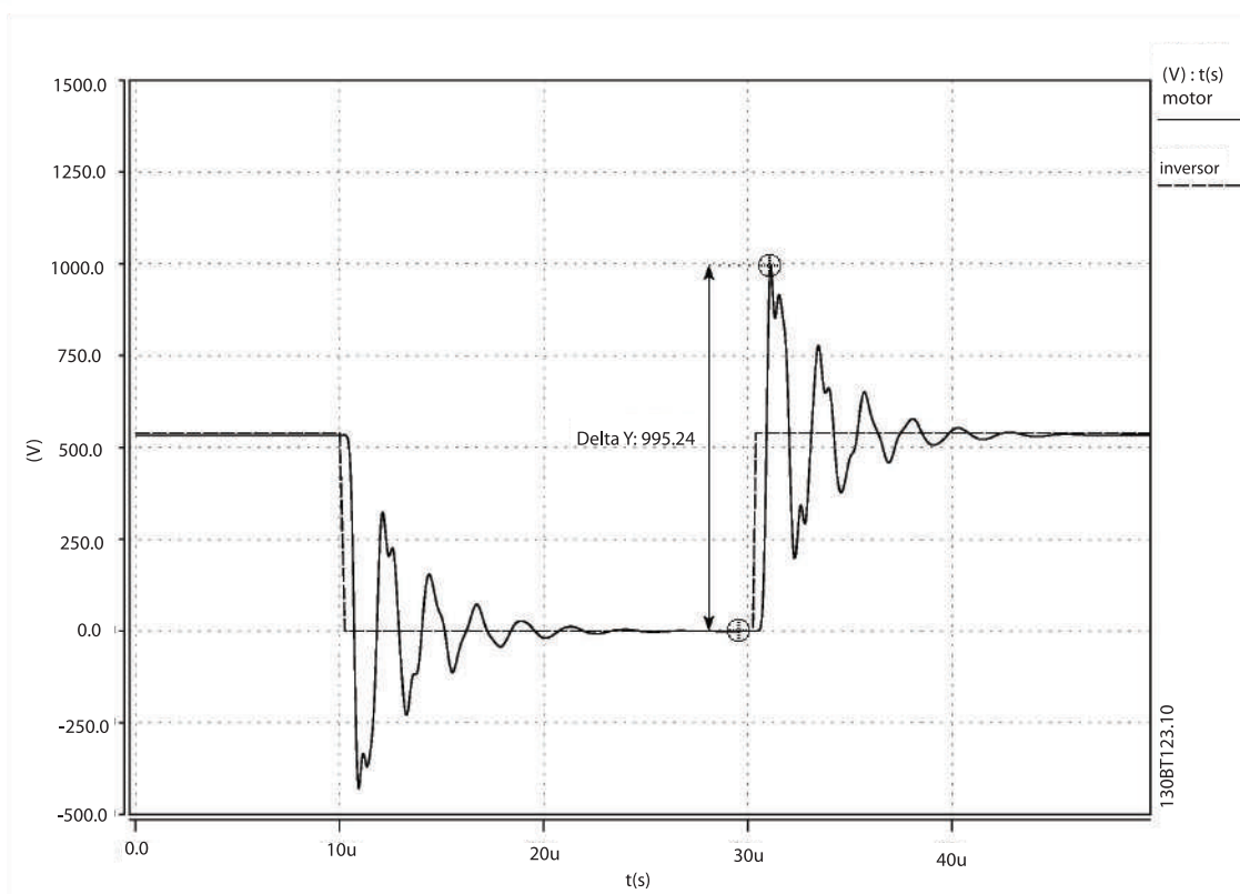
Ilustración 3.1 Ejemplo de tensión de salida del convertidor (línea de puntos) y tensión del terminal del motor después de 200 m de cable (línea continua).
