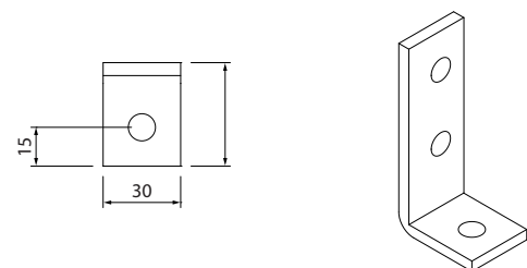
Ilustración 5.15 Kit de terminal en forma de L 130B3137
