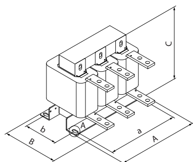
Ilustración 5.13 IP00 con montaje en suelo
