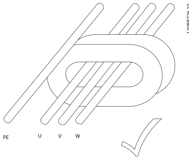
Ilustración 5.1 Instalación correcta
