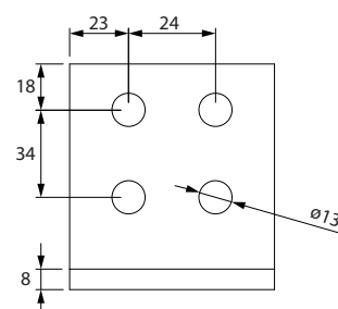
Ilustración 5.16 Kit de terminal en forma de L 130B3138
