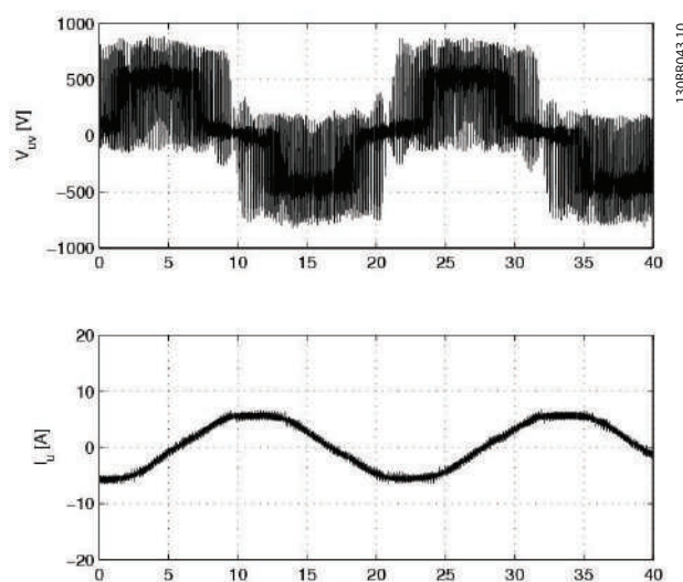
Ilustración 3.10 Con filtro du/dt
