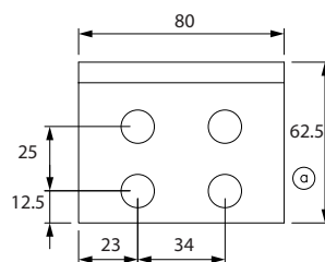
Ilustración 5.17 Kit de terminal en forma de L 130B3139
