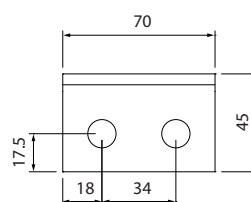
Ilustración 5.16 Kit de terminal en forma de L 130B3138
