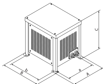
Ilustración 5.14 IP23 con montaje en suelo
