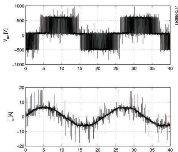
Ilustración 3.9 Sin filtro
