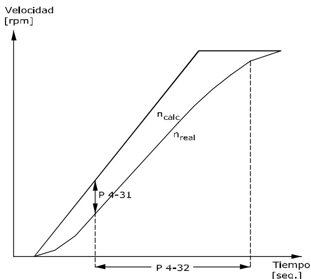
Ilustración 4.8 Error de velocidad en realim. del motor
