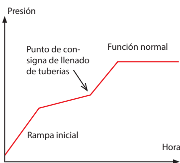
Modo Llenado de Tuberías para evitar golpes de ariete
