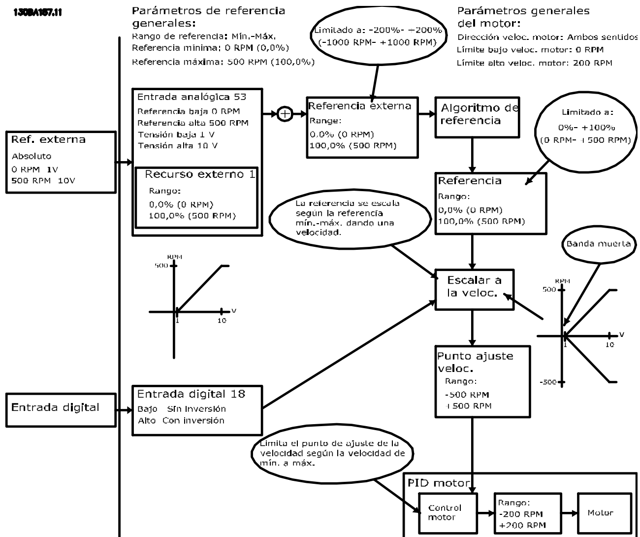
Ilustración 3.21 Referencia positiva con banda muerta, entrada digital para disparar inversión
