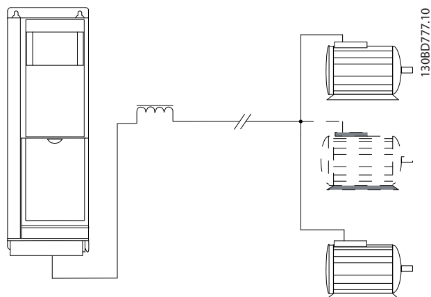
Ilustración 9.53 Cables paralelos con carga
