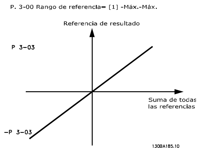
Ilustración 3.15 Referencia resultante
