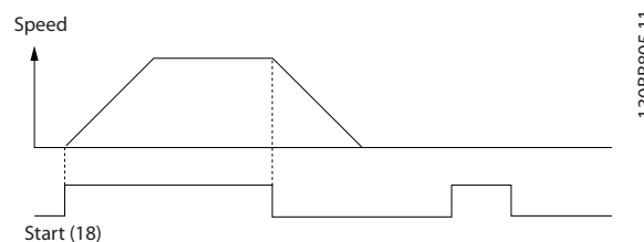
Ilustración 10.1 Arranque / parada con desconexión segura de par
