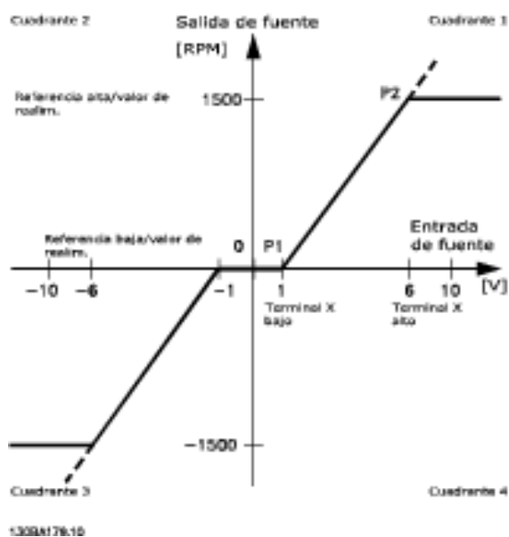
Ilustración 3.19 Banda muerta
