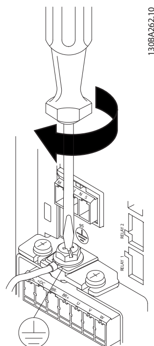
Ilustración 9.18 Apriete del cable de conexión a tierra
