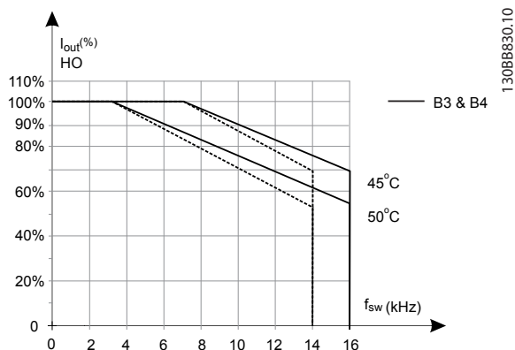
Ilustración 6.8 Reducción de potencia de I_{salida} para diferentes T_{AMB, MÁX.} para tipos de protección B3 y B4, utilizando AVM de 60° en modo de sobrecarga alto (160 % por encima del par)
