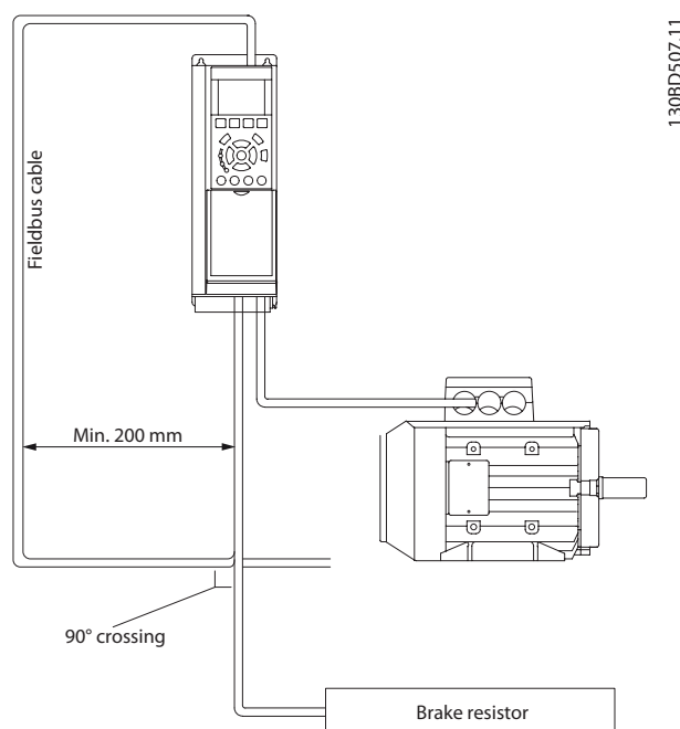
Ilustración 12.4 Enrutado de los cables
