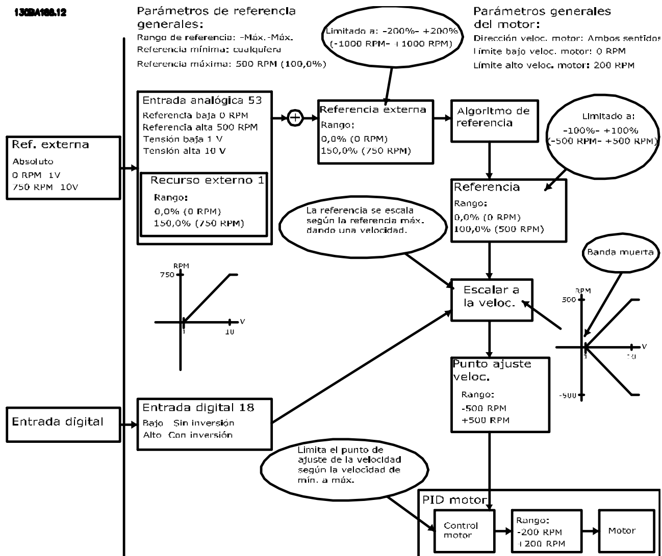
Ilustración 3.22 Referencia positiva con banda muerta, entrada digital para disparar inversión. Reglas de bloqueo
