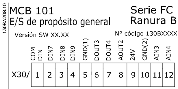
Ilustración 11.1 Opción MCB 101
