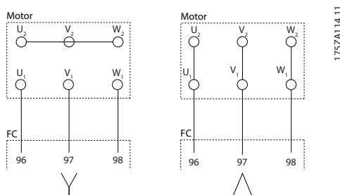
Ilustración 9.29 Conexiones en estrella y en triángulo
