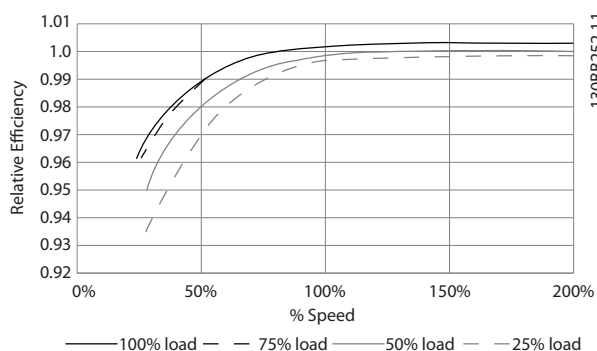
Ilustración 6.35 Curvas de rendimiento típico
