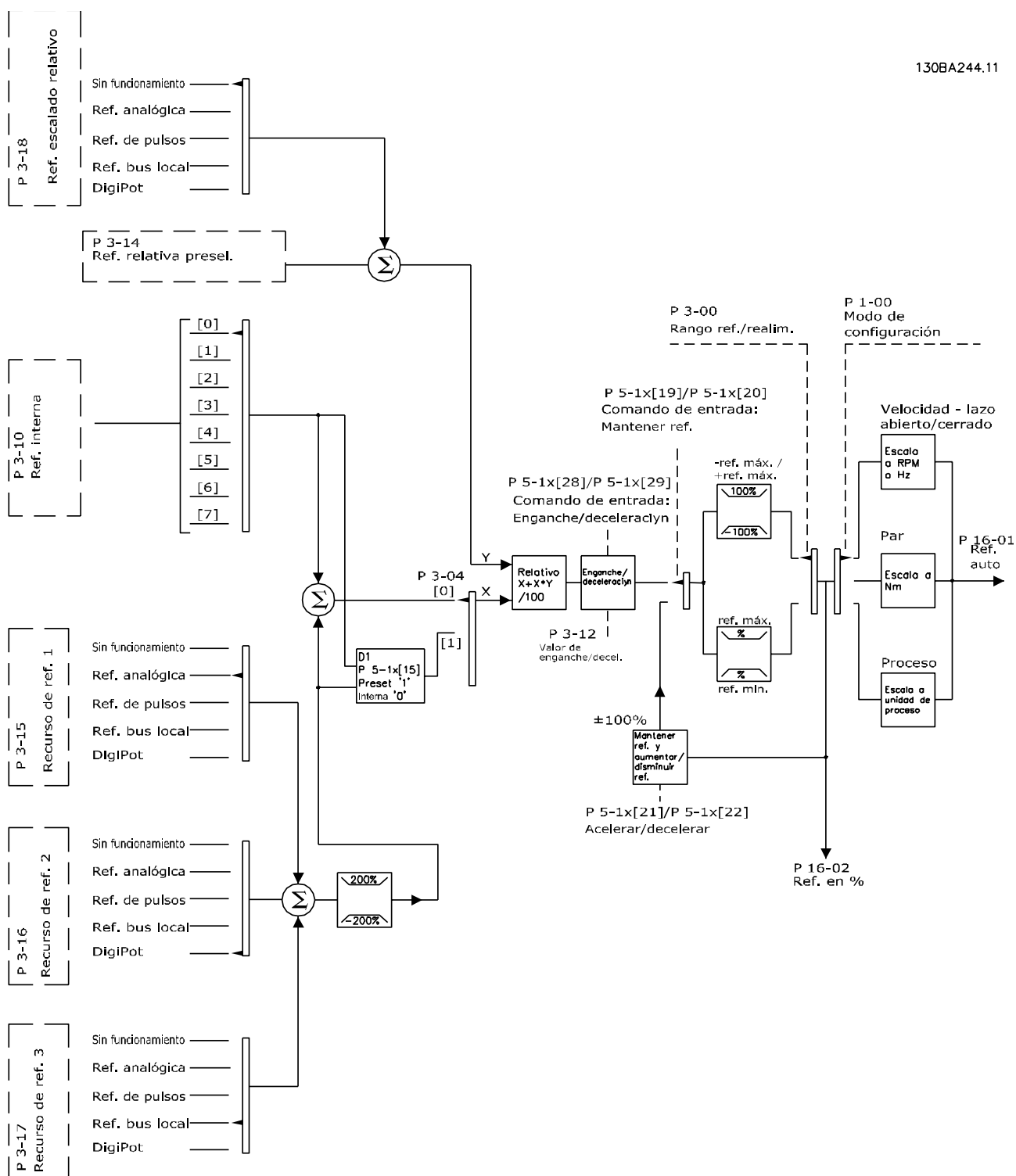
Ilustración 3.13 Referencia remota
