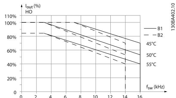
Ilustración 6.6 Reducción de potencia de I_{salida} para diferentes T_{AMB} , MÁX. para tipos de protección B1 y B2, utilizando AVM de 60° en modo de sobrecarga alto (160 % por encima del par)
