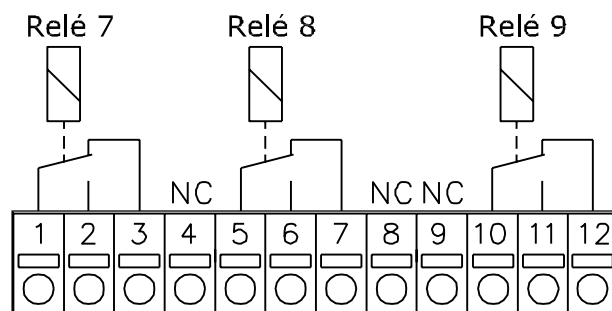
Ilustración 11.10 Relés
