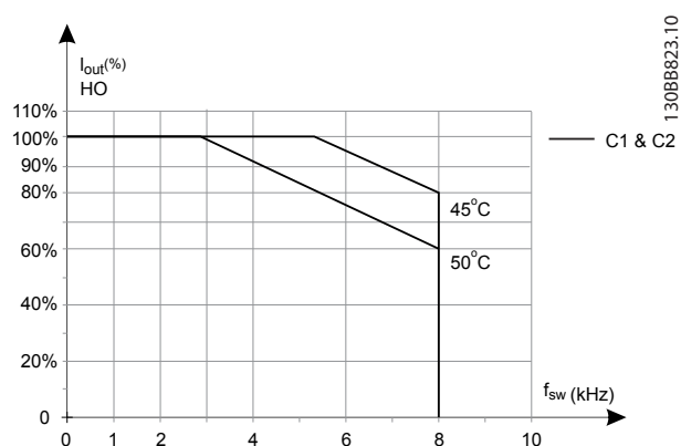
Ilustración 6.29 Reducción de potencia de la intensidad de salida con frecuencia de conmutación y temperatura ambiente para convertidores de frecuencia de 600 V, tipos de protección C, AVM de 60°, HO
