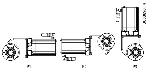
Ilustración 4.8 OneGearDrive
