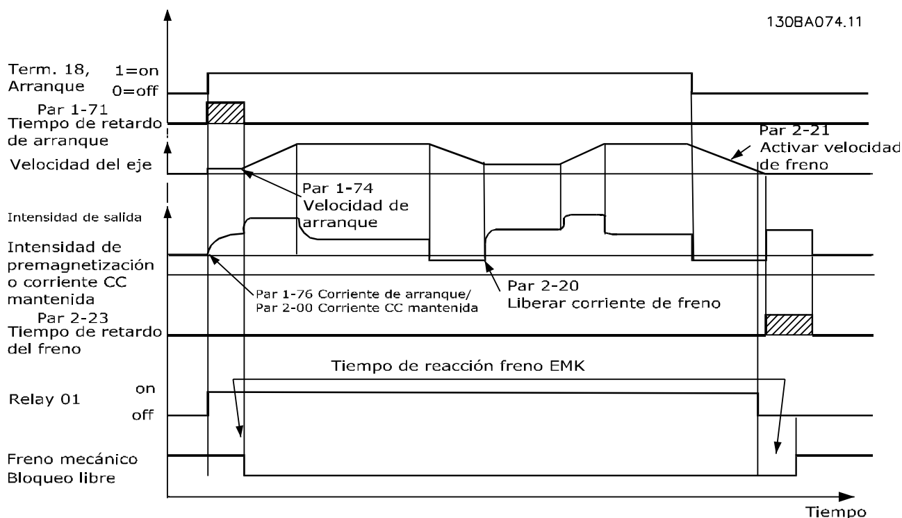
Ilustración 4.2 Freno mecánico
