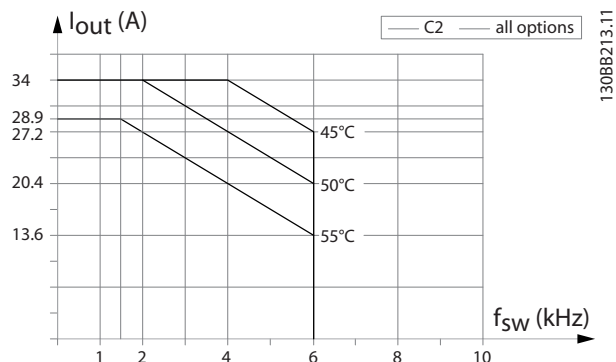
Ilustración 6.32 Reducción de potencia de la intensidad de salida con frecuencia de conmutación y temperatura ambiente para tipo de protección C2, AVM de 60°. Nota: El gráfico muestra la intensidad como un valor absoluto y es válido tanto para sobrecarga normal como alta
