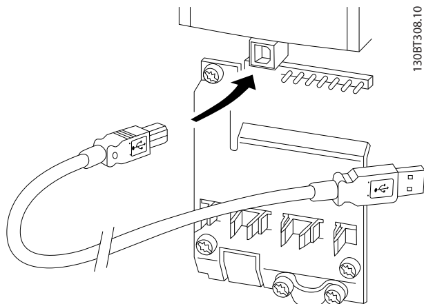
Ilustración 9.48 Conexión USB
