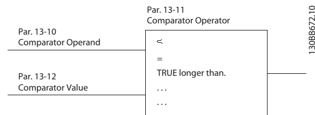
Ilustración 4.6 Comparadores
