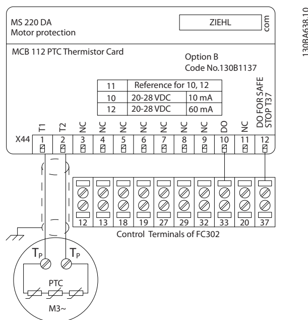
Ilustración 11.15 Instalación del MCB 112
