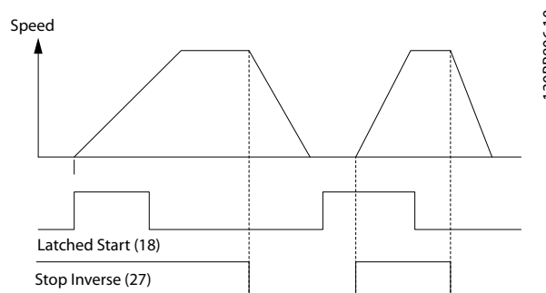
Ilustración 10.2 Arranque de impulsos / parada inversa
