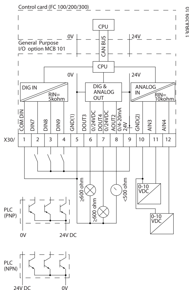
Ilustración 11.2 Diagrama básico
