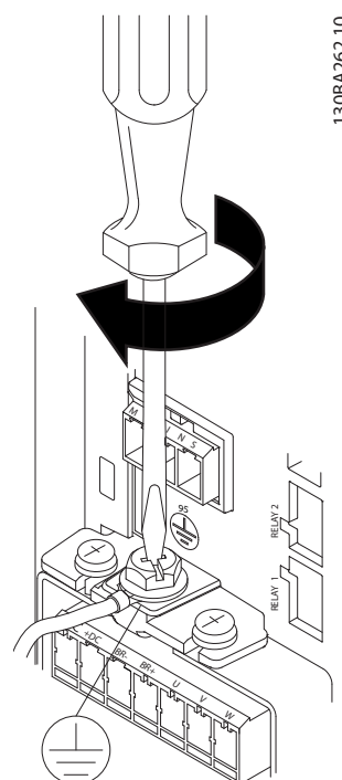
Ilustración 9.18 Apriete del cable de conexión a tierra
