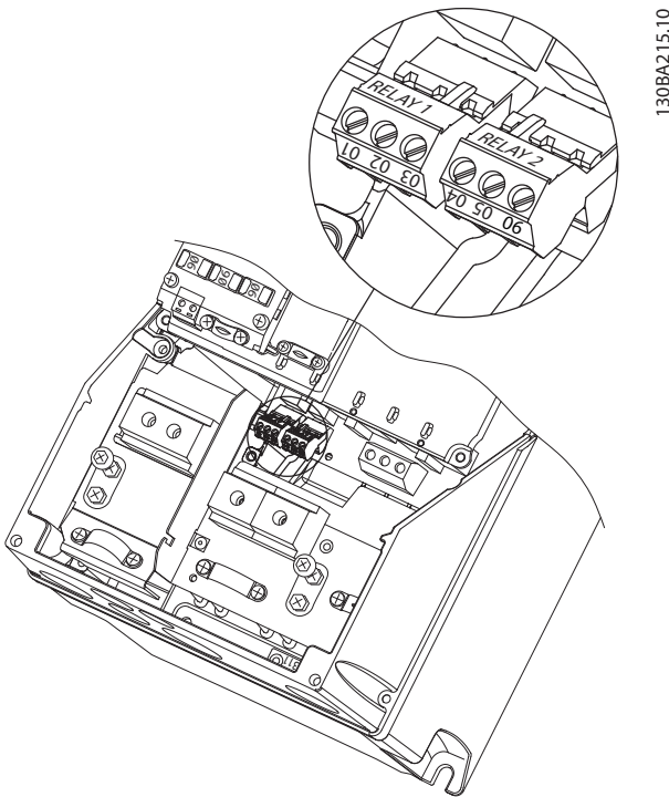
Ilustración 9.44 Terminales para conexión del relé (Tipos de protección A5, B1 y B2).
