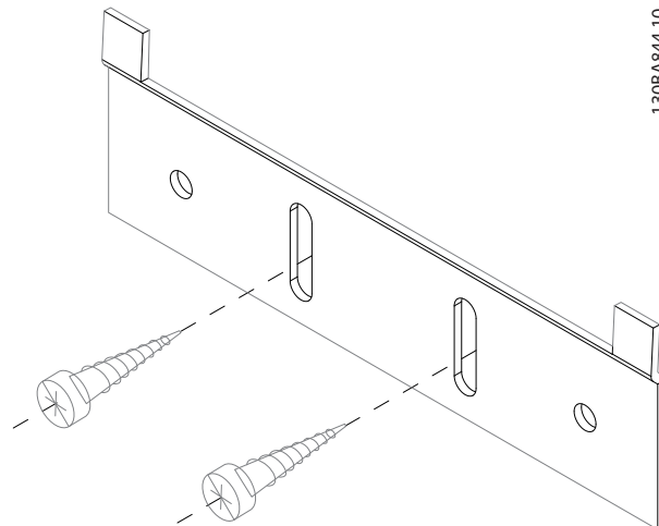
Ilustración 11.30 Soporte inferior
