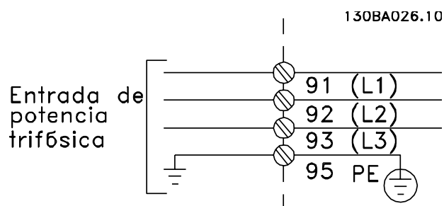
Ilustración 9.16 Conexión de red
