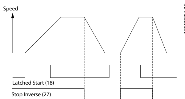
Ilustración 10.2 Arranque de impulsos / parada inversa
