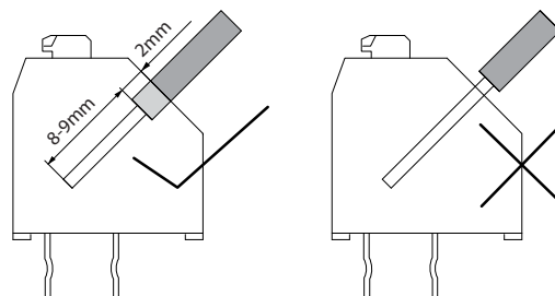
Ilustración 11.11 Inserción correcta de los cables
