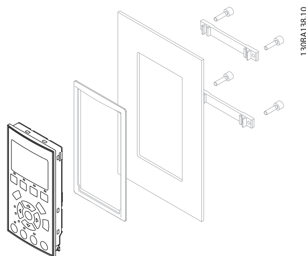
Ilustración 11.27 Kit LCP con LCP gráfico, sujetores, cable de 3 m y junta.
