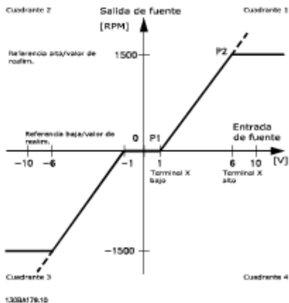
Ilustración 3.19 Banda muerta
