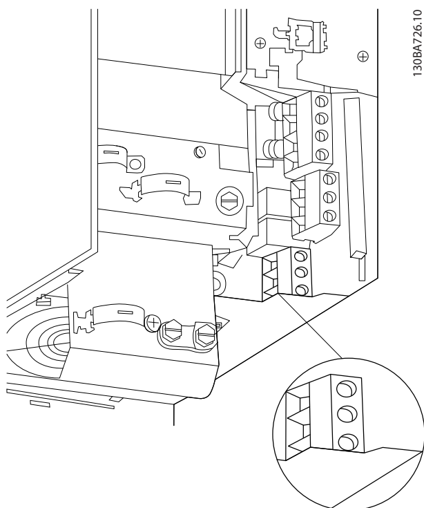
Ilustración 9.33 Conexión del motor para protección B3
