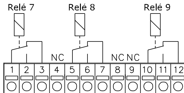
Ilustración 11.10 Relés
