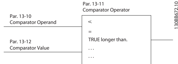
Ilustración 4.6 Comparadores
