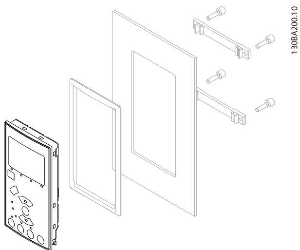
Ilustración 11.28 Kit LCP con LCP numérico, sujetones y junta. N.º de pedido 130B1114
