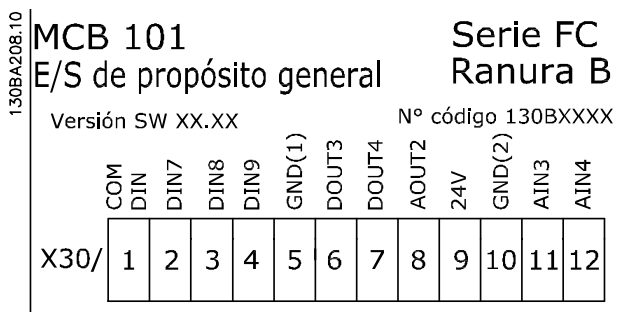
Ilustración 11.1 Opción MCB 101
