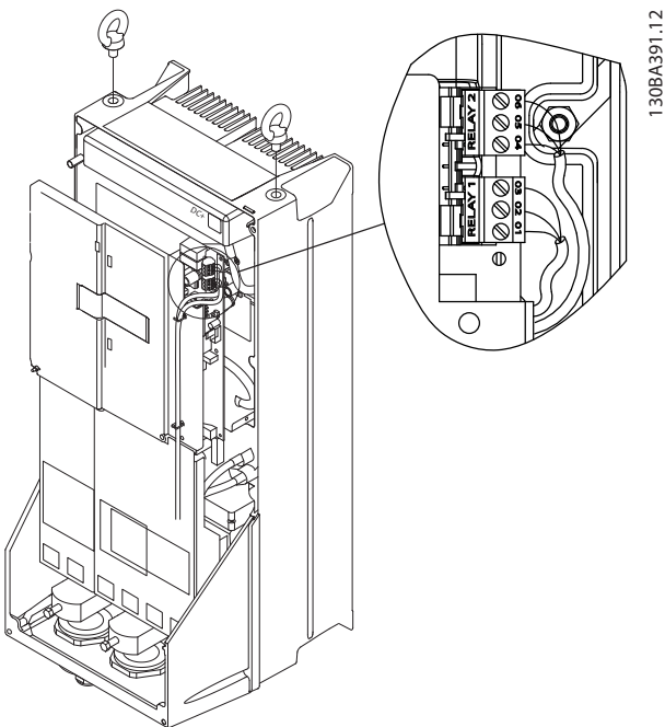
Ilustración 9.43 Terminales para conexión del relé (Tipos de protección C1 y C2).
