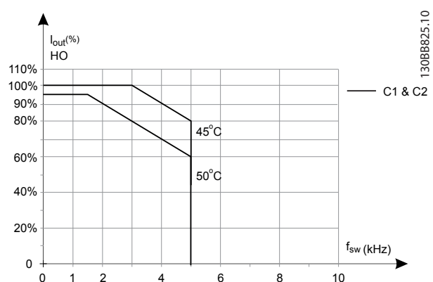
Ilustración 6.31 Reducción de potencia de la intensidad de salida con frecuencia de conmutación y temperatura ambiente para convertidores de frecuencia de 600 V, tipos de protección C; SFAVM, HO
