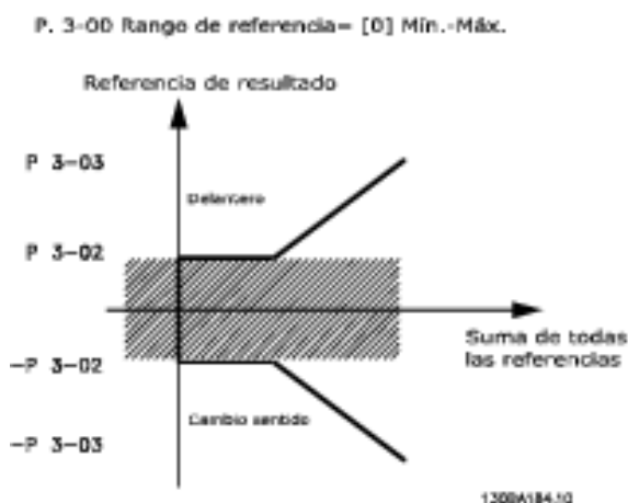
Ilustración 3.14 Relación entre la referencia resultante y la suma de todas las referencias
