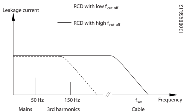
Ilustración 9.39 Contribuciones principales a la corriente de fuga
