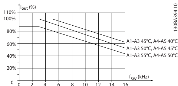
Ilustración 6.4 Reducción de potencia de I_{salida} para diferentes T_{AMB} , MÁX. para tipo de protección A, utilizando AVM de 60° y un cable de motor de 10 m como máximo
