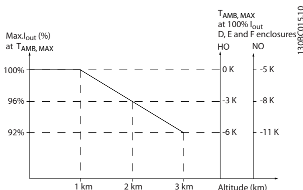
Ilustración 5.2 Reducción de potencia de la intensidad de salida en relación con la altitud a T_{AMB, MAX} para tamaños de bastidor D3h.
