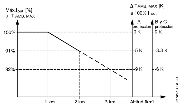
Ilustración 5.1 Reducción de potencia de la intensidad de salida en relación con la altitud a T_{AMB, MAX} para tamaños del bastidor A, B y C. Para altitudes superiores a 2000 m, póngase en contacto con (Danfoss) en relación con PELV.
