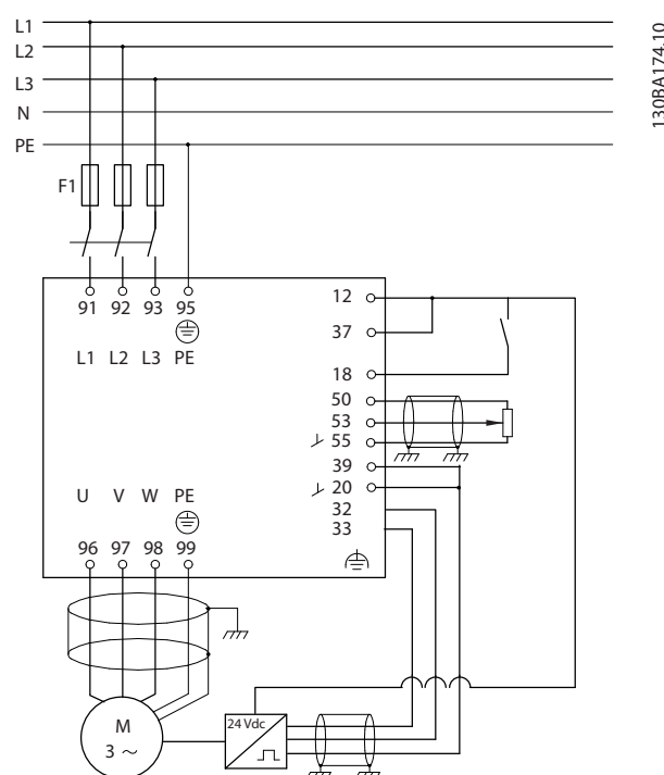
Ilustración 10.7 Ejemplo: conexión del control de velocidad
