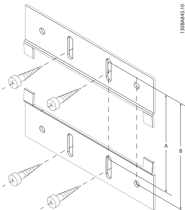
Ilustración 3.39 Soporte superior
