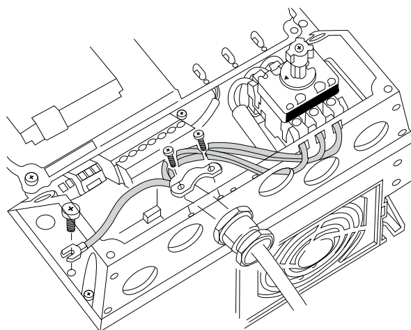
Ilustración 8.3 Conexión de red y toma de tierra sin desconector (en variantes S2 de tamaño de protección B2, el bloque extra de terminales debe usarse para la conexión de red).
