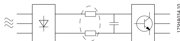
Ilustración 3.3 Bobinas del circuito intermedio
