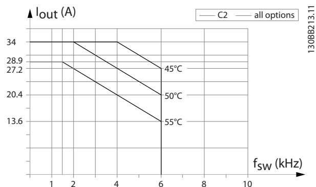
Ilustración 5.21 Reducción de potencia de la intensidad de salida con frecuencia de conmutación y temperatura ambiente para tamaño de protección C2, AVM de 60°.
