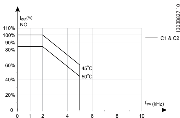
Ilustración 5.20 Reducción de potencia de la intensidad de salida con frecuencia de conmutación y temperatura ambiente para convertidores de frecuencia de 600 V, tamaño de protección C; SFAVM, NO
