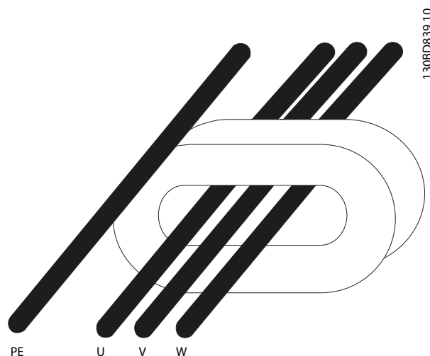
Ilustración 3.30 Núcleo HF-CM con las fases del motor
