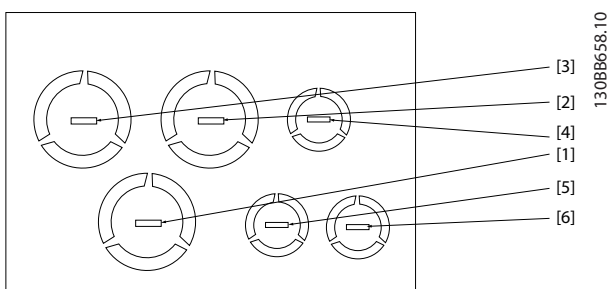
Ilustración 8.32 Tamaño de protección B2, IP55 Orificios roscados para prensacables
