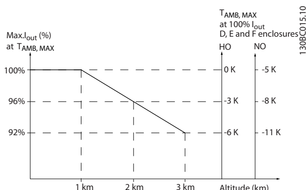
Ilustración 5.2 Reducción de potencia de la intensidad de salida frente a la altitud a T_{AMB, MÁX.} para tamaño de protección D3h.
