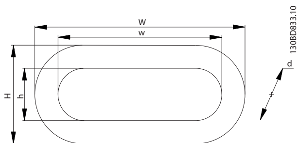
Ilustración 6.4 Núcleo HF-CM
