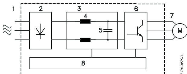
Ilustración 2.9 Diagrama de bloques de convertidor de frecuencia
