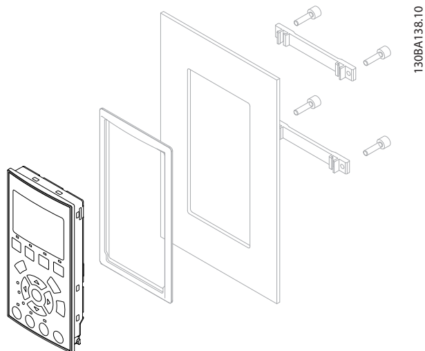
Ilustración 3.35 Kit LCP con LCP gráfico, sujetiones, cable de 3 m y junta.
