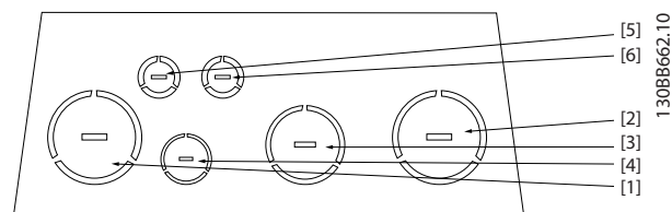
Ilustración 8.34 Tamaño de protección C1, IP21
