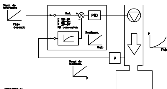
Ilustración 2.17 Conversión de realimentación
