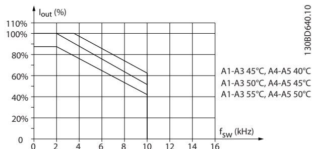
Ilustración 5.6 Reducción de potencia de I_{sal} para diferentes T_{AMB, MÁX.} para tipos de protección A, con SFAVM y un cable de motor de 10 m como máximo
