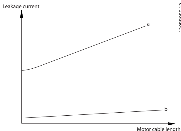
Ilustración 3.6 La longitud del cable de motor y el tamaño de potencia influyen en la corriente de fuga. Potencia a > potencia b
