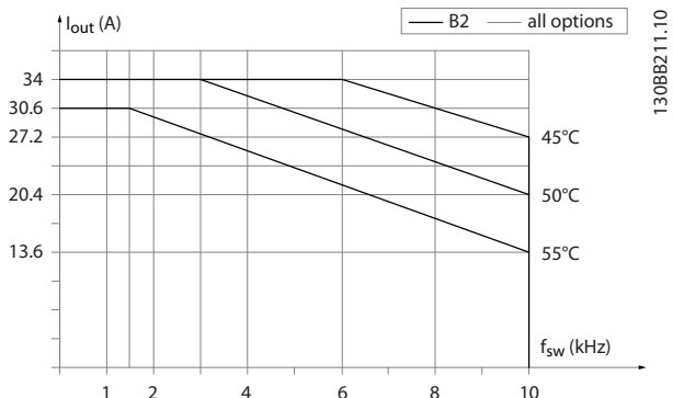
Ilustración 5.13 Reducción de potencia de la intensidad de salida con frecuencia de conmutación y temperatura ambiente para tamaños de protección B2 y B4, AVM de 60°.
