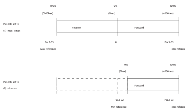
Ilustración 3.58 Referencia y MAV
