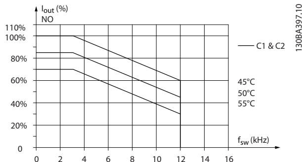
Ilustración 5.15 Reducción de potencia de I_{sal} para diferentes T_{AMB, MÁX.} para tamaños de protección C1 y C2 con AVM de 60° en modo de sobrecarga normal (110 % por encima del par)
