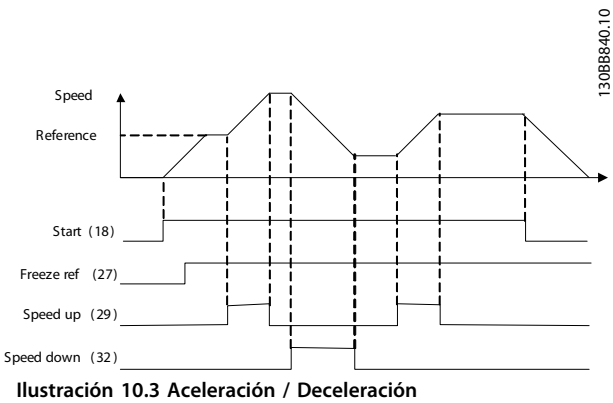
Ilustración 10.3 Aceleración / Deceleración
