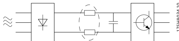
Ilustración 5.4 Bobinas del circuito intermedio
