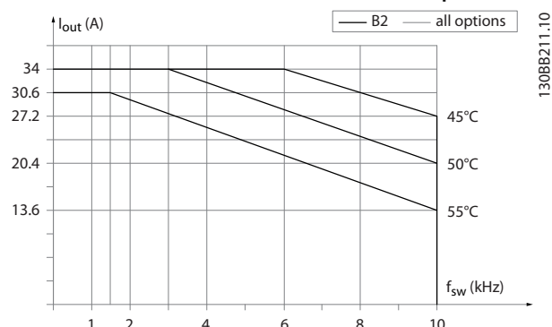
Ilustración 6.18 Reducción de potencia de la intensidad de salida con frecuencia de conmutación y temperatura ambiente para tipos de protección B2 y B4, AVM de 60°. Nota: El gráfico muestra la intensidad como un valor absoluto y es válido tanto para sobrecarga normal como alta.
