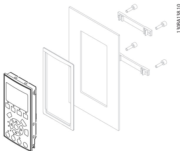
Ilustración 11.27 Kit LCP con LCP gráfico, sujetaciones, cable de 3 m y junta.
