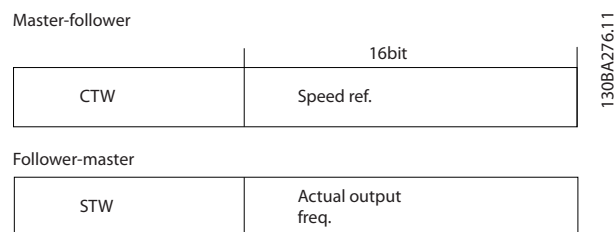
Ilustración 12.18 Frecuencia de salida real (MAV)
