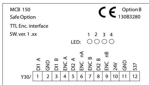
Ilustración 11.20 MCB 150
