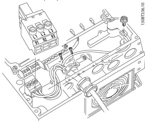
Ilustración 9.21 Conexión a la red y a tierra sin desconector
