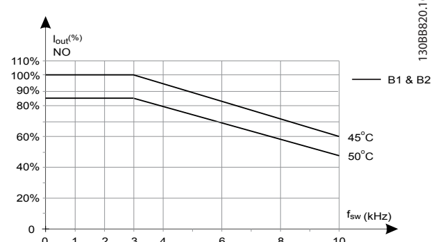
Ilustración 5.11 Reducción de potencia de la intensidad de salida con frecuencia de conmutación y temperatura ambiente para convertidores de frecuencia de 600 V, tamaño de protección B, 60 AVM, NO
