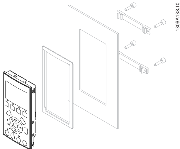
Ilustración 3.35 Kit LCP con LCP gráfico, sujeciones, cable de 3 m y junta.
