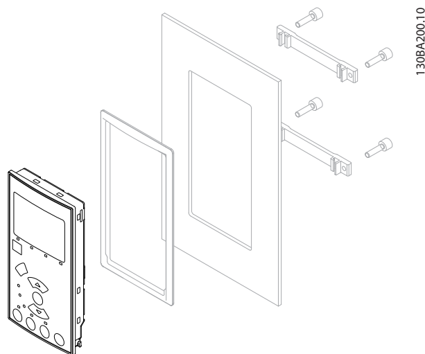
Ilustración 3.36 Kit LCP con LCP numérico, sujeciones y junta. Número de pedido 130B1114
