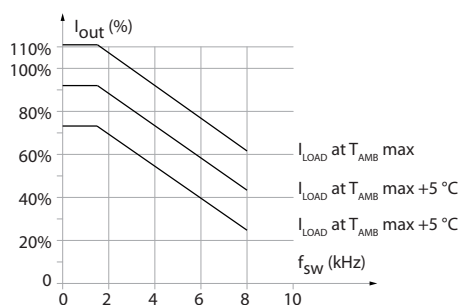
Ilustración 5.23 Reducción de potencia de la intensidad de salida con frecuencia de conmutación y temperatura ambiente para tamaño de protección C3
