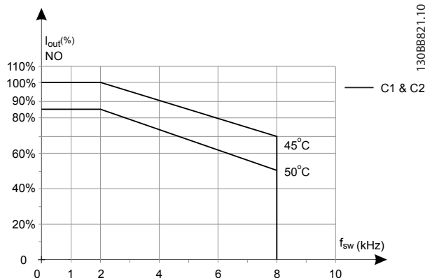
Ilustración 5.19 Reducción de potencia de la intensidad de salida con frecuencia de conmutación y temperatura ambiente para convertidores de frecuencia de 600 V, tamaño de protección C, 60 AVM, NO
