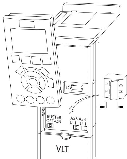
Ilustración 4.11 Ubicación de los conmutadores de los terminales 53 y 54
