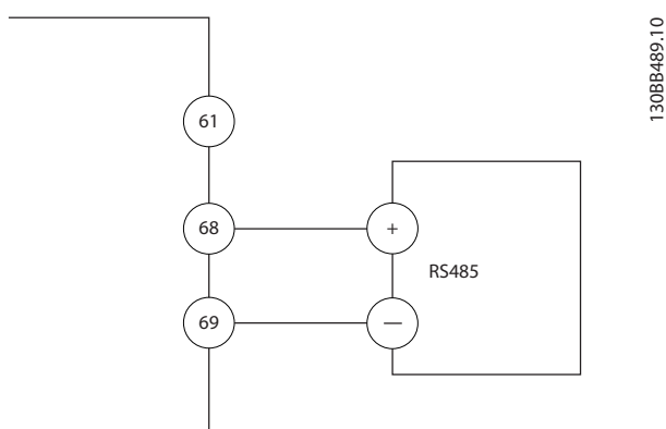
Ilustración 4.12 Diagrama de cableado de comunicación serie
