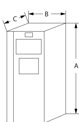
Ilustración 9.4 Estándar con kit IP21/UL/Tipo 1
