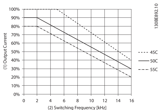
Ilustración 7.5 Curva de reducción de potencia K3T4
