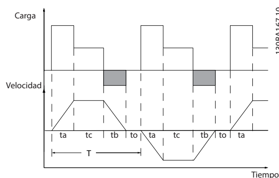
Ilustración 2.33 Ciclo de frenado típico
