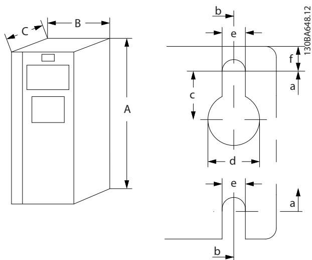
Ilustración 7.16 Agujeros de montaje superiores e inferiores
