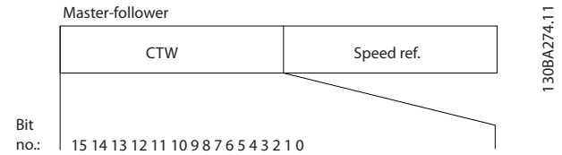
Ilustración 5.13 Código de control según el perfil FC
