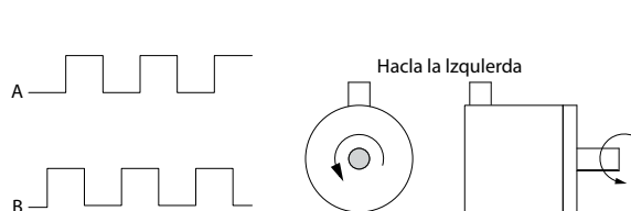
Ilustración 3.2 Codificador incremental de 24 V con una longitud máxima del cable de 5 m (16,4 ft)
