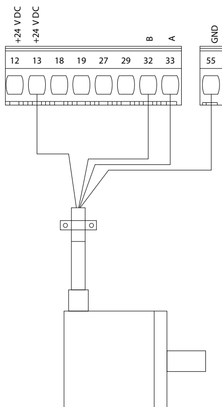
Ilustración 3.1 Encoder 24 V
