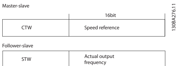
Ilustración 5.15 Frecuencia real de salida (MAV)
