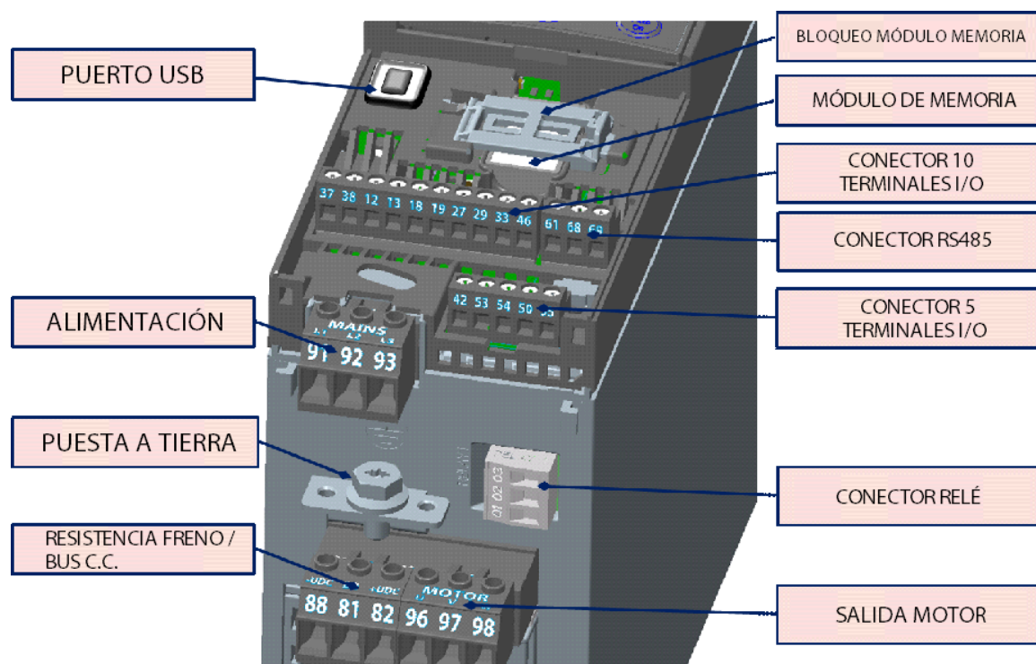
Fig.23: Conexiones FC-280
