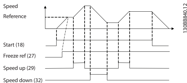
Ilustración 3.4 Aceleración/desaceleración
