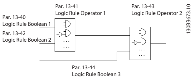
Ilustración 2.37 Reglas lógicas
