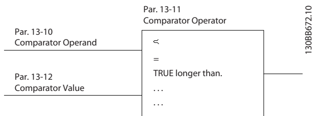
Ilustración 2.36 Comparadores
