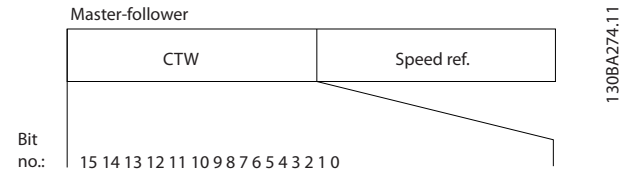
Ilustración 5.13 Código de control según el perfil FC
