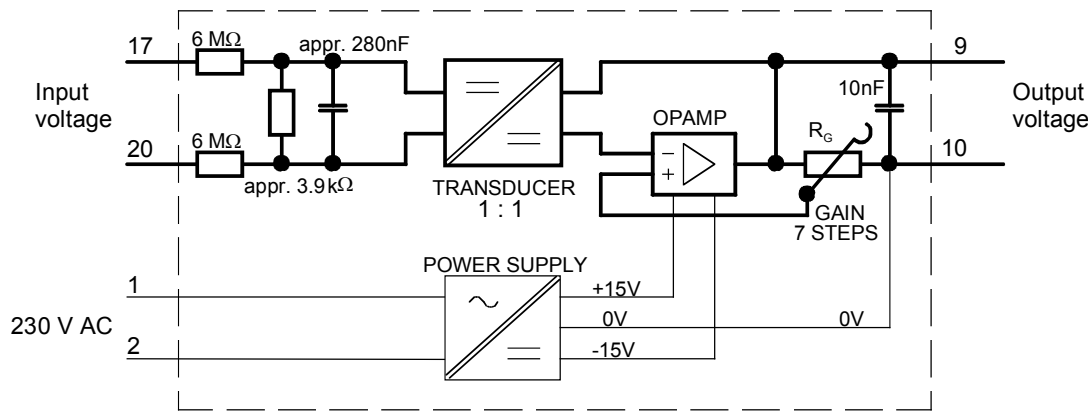
Diagrama del circuito principal del transductor CC-CC A92
