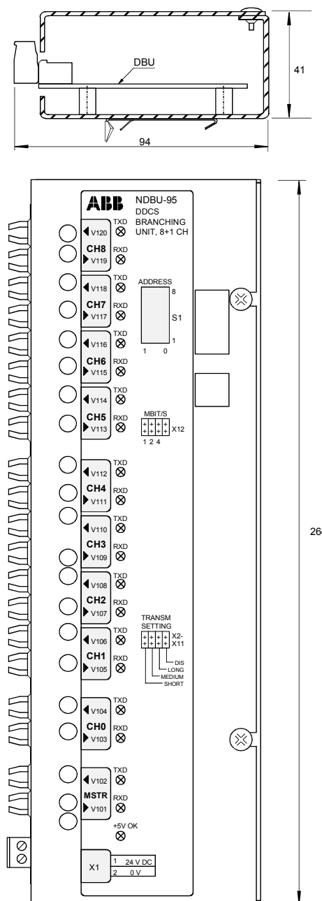
Disposición de la unidad de distribución NDBU-95
