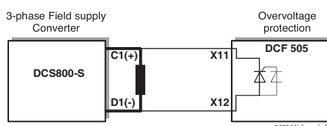
Carga simple con DCS800-S01 y protección contra sobretensiones 2-Q DCF505
