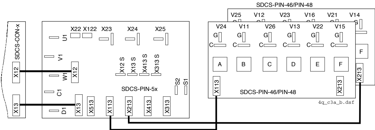
Tarjeta transformadora de pulsos SDCS-PIN-46/PIN-48 Disposición de la tarjeta transformadora de pulsos SDCS-PIN-46/PIN-48
