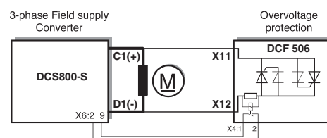
Alimentación de excitación del motor con DCS800-S02 y protección contra sobretensiones 4-Q DCF506
