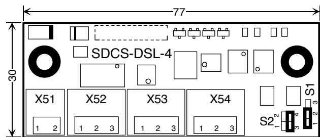
DSL-4_drw.dsf
