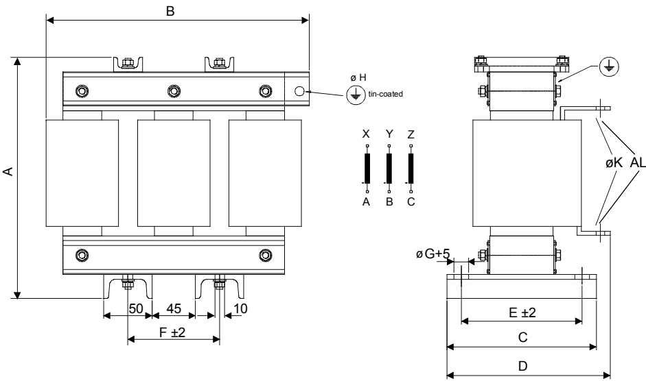
Reactancias de línea tipo ND 409 ... ND 413
