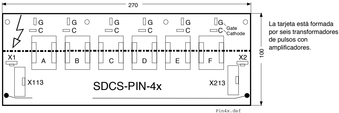
Tarjeta transformadora de pulsos SDCS-PIN-46/PIN-48 Disposición de la tarjeta transformadora de pulsos SDCS-PIN-46/PIN-48
