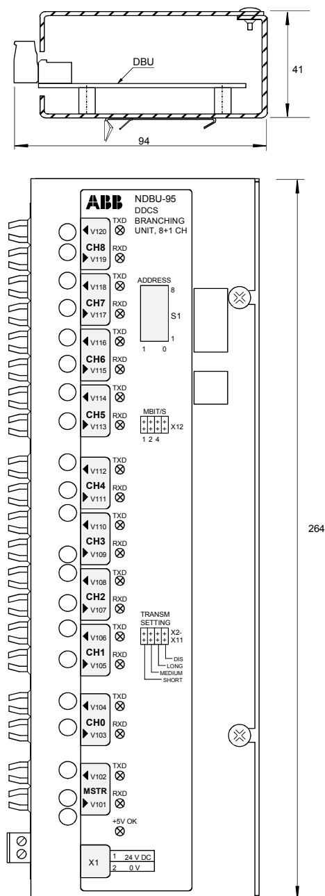
Disposición de la unidad de distribución NDBU-95
