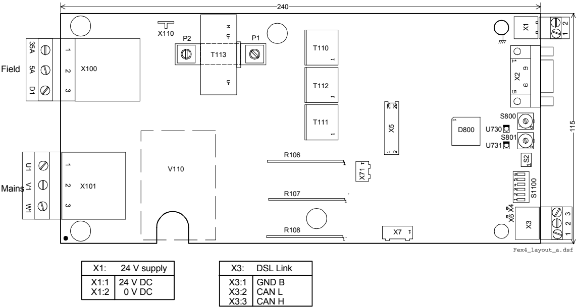
Disposición de la tarjeta SDCS-FEX-4
