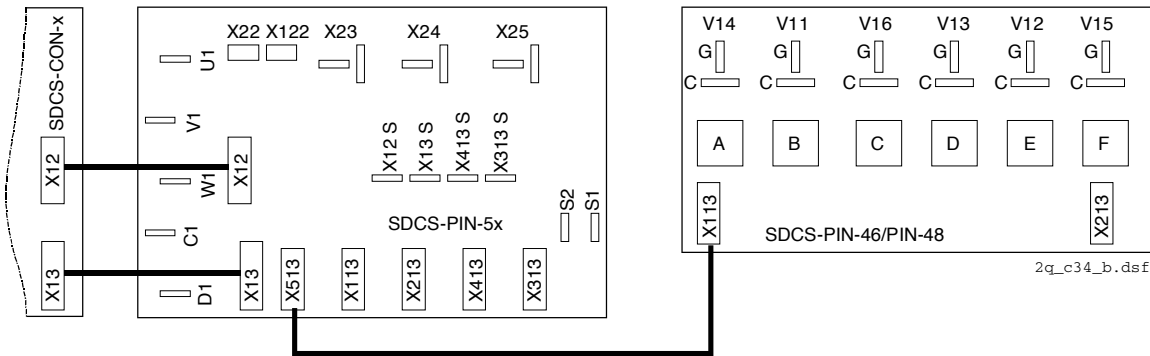
Aplicación de 4 cuadrantes, sin tiristores en paralelo - Tipo de estructura D5/D6/D7
