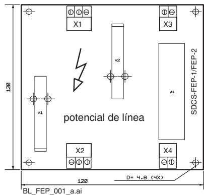
Disposición de SDCS-FEP-1/FEP-2.
