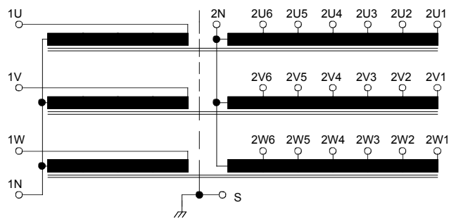
Esquema de principios del transformador T90
