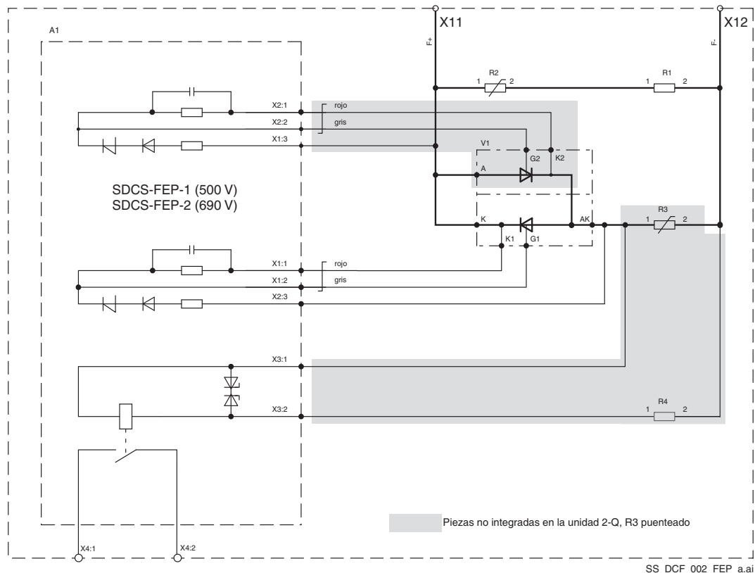
Protección contra sobretensiones DCF505/DCF506.
