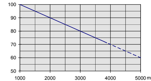
Reducción de intensidad al % de la intensidad nominal del convertidor
