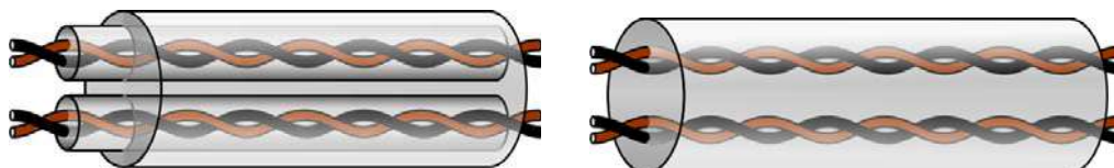
A: Cable de par trenzado, apantallamiento doble.
