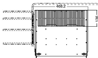
Ejemplo de conexión en el lado derecho
