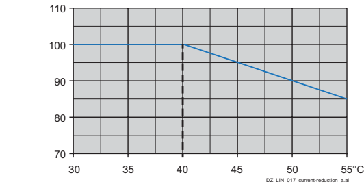
Reducción de intensidad al % de la intensidad nominal del convertidor
