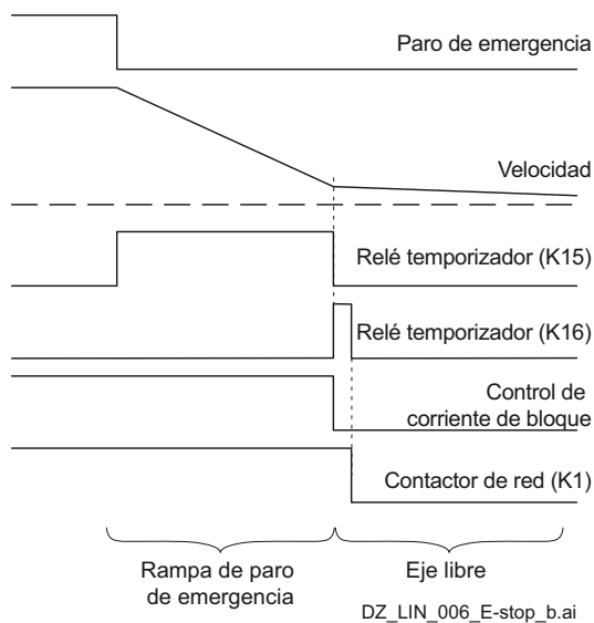
Reacción de paro de emergencia
