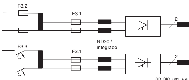
Configuraciones para circuito de campo.
