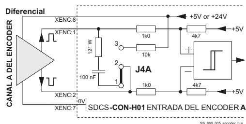
Ajustes de puentes para encoders diferenciales conectados a SDCS-CON-H01
