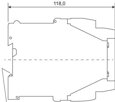
Montaje a presión para rail de 35 mm DIN EN 50 022
