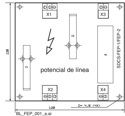
Disposición de SDCS-FEP-1/FEP-2.
